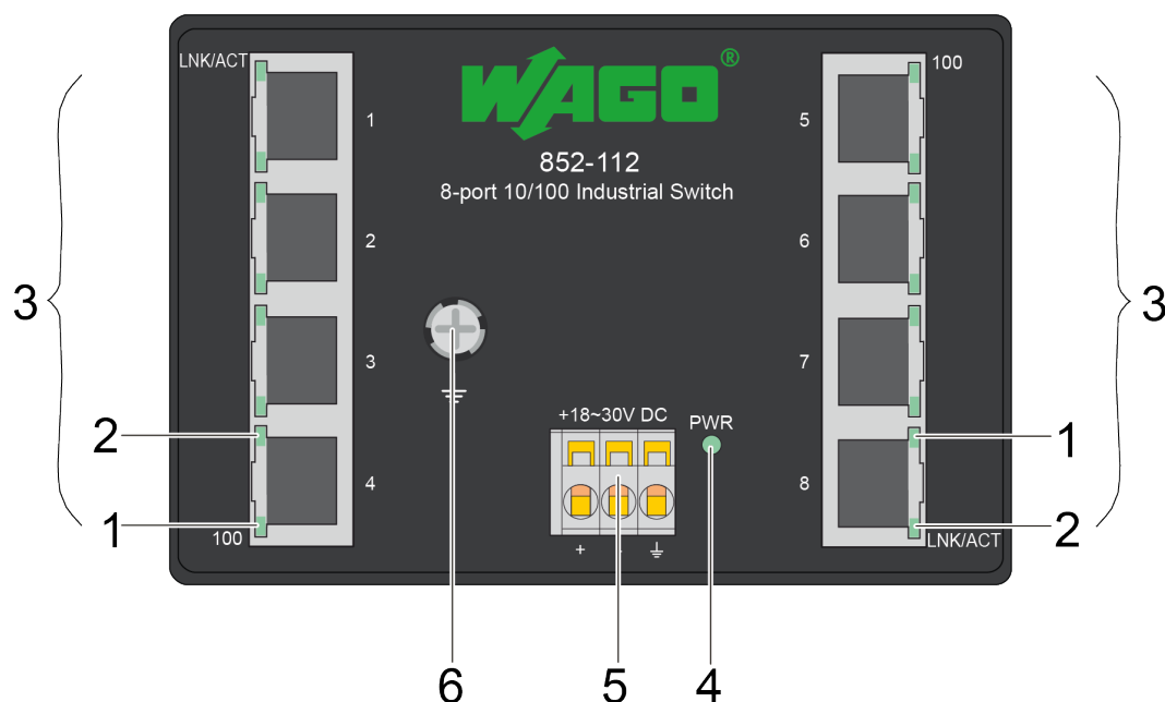
Abbildung 1: Frontansicht des Industrial-ECO-Switches
