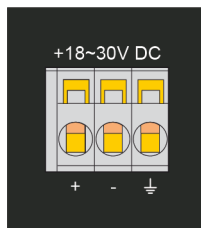
Abbildung 3: Anschluss Spannungsversorgung (PWR)
