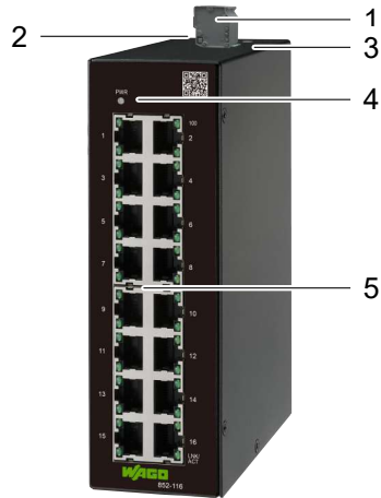
Abbildung 1: Frontansicht
