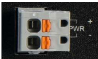
Abbildung 3: Spannungsversorgungsanschluss
