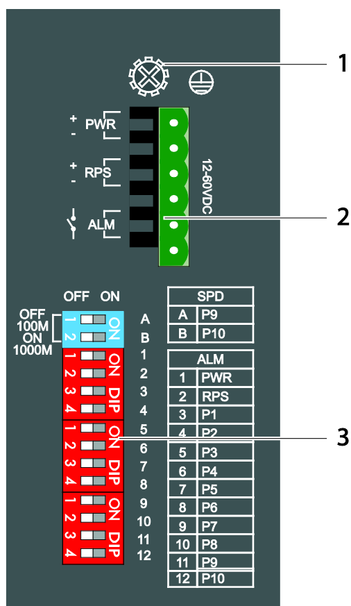
Abbildung 2: Draufsicht des Industrial-Managed-Switches (Beispiel)
