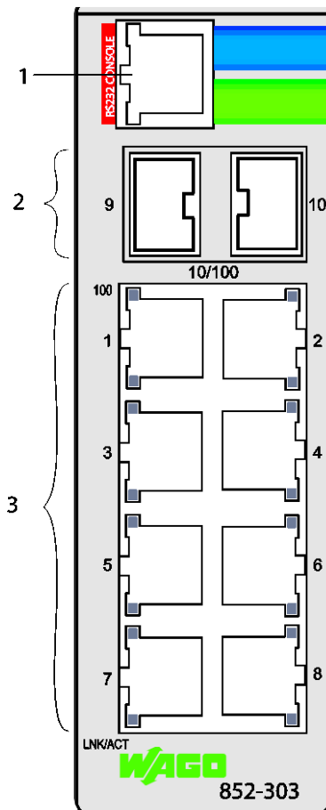
Abbildung 4: Netzwerkanschlüsse
