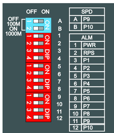
Abbildung 7: DIP-Schalter (Beispiel)
