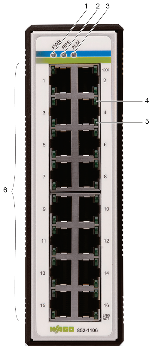
Abbildung 1: Frontansicht des Industrial-Switches (gültig auch für Version 852-1106/010-000)
