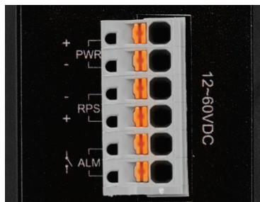
Abbildung 4: Anschluss Spannungsversorgung (PWR/RPS)
