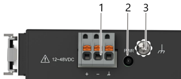
Abbildung 2: Draufsicht des Industrial-Eco-Switches
