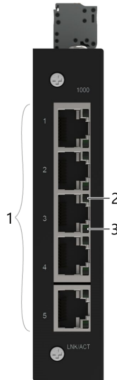
Abbildung 1: Frontansicht des Industrial-Eco-Switches
