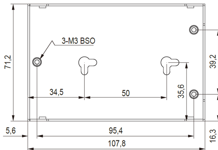
Abbildung 9: Abmaße der Befestigungslöcher
