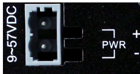
Abbildung 4: Anschluss Spannungsversorgung (PWR)
