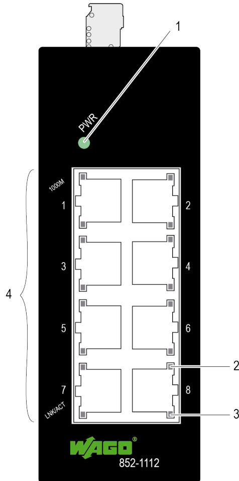
Abbildung 1: Frontansicht des Industrial-Eco-Switches
