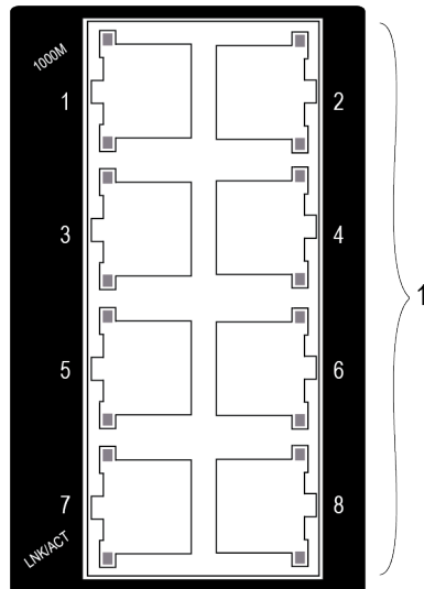
Abbildung 5: Netzwerkanschlüsse
