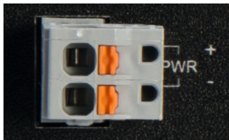
Abbildung 3: Spannungsversorgungsanschluss
