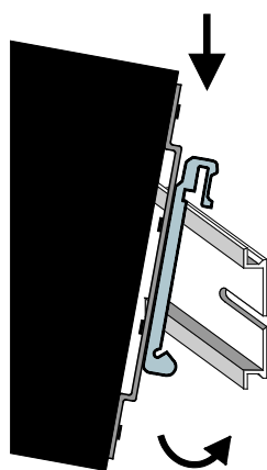
Abbildung 9: Aufrasten auf Tragschiene
