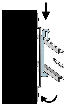
Abbildung 10: Entfernen von Tragschiene
