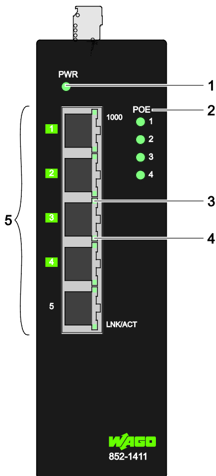
Abbildung 1: Frontansicht des Industrial-Eco-Switches
