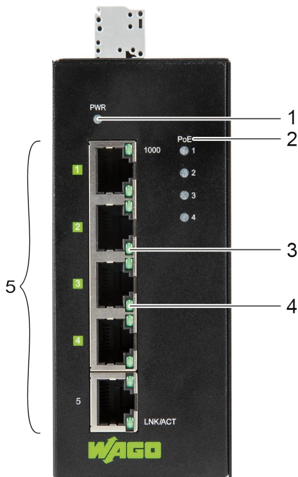
Abbildung 1: Frontansicht des Industrial-Eco-Switches
