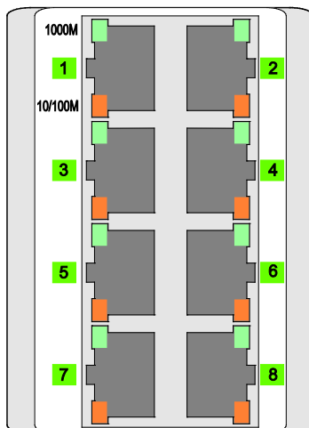
Abbildung 6: Anschluss-LEDs
