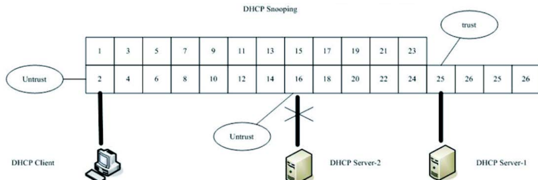
Abbildung 24: DHCP Snooping
