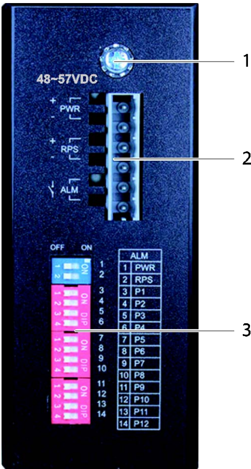
Abbildung 2: Draufsicht des Industrial-Managed-Switches
