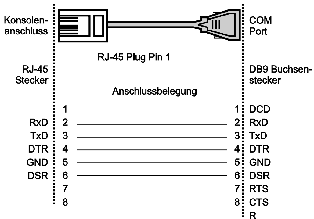
Abbildung 123: Anschlussbelegung RJ-45 zu DB9
