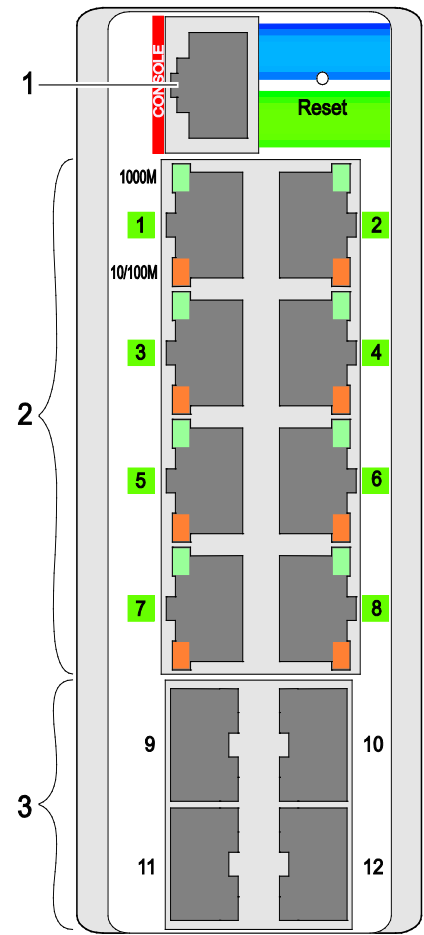
Abbildung 4: Netzwerkanschlüsse
