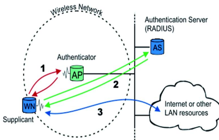
Abbildung 25: IEEE 802.1X
