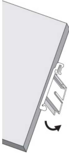
Abbildung 6: Produkt auf Tragschiene montieren
