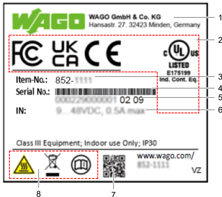
Abbildung 2: Typenschild (Beispiel)
