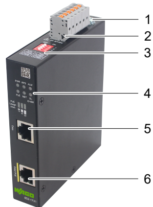
Abbildung 1: Frontansicht
