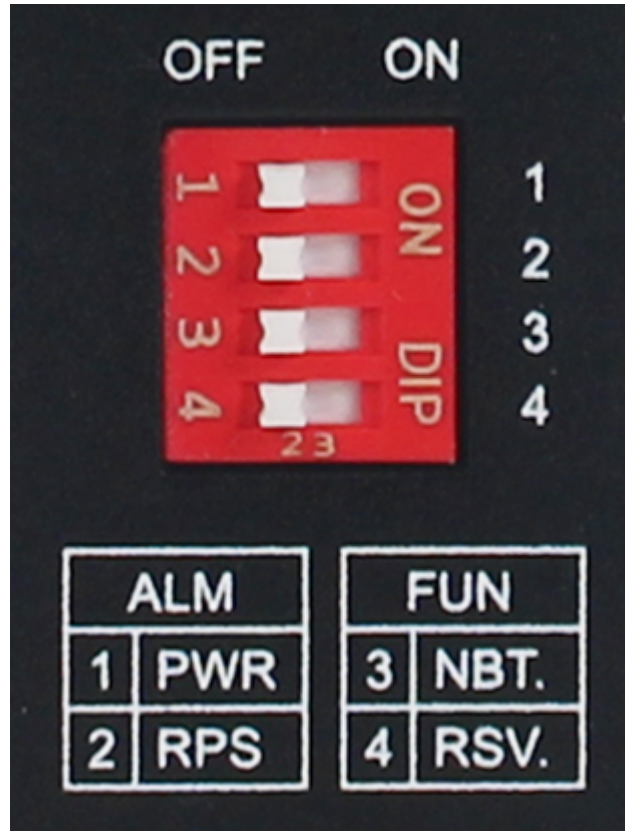
Abbildung 6: DIP-Schalter
