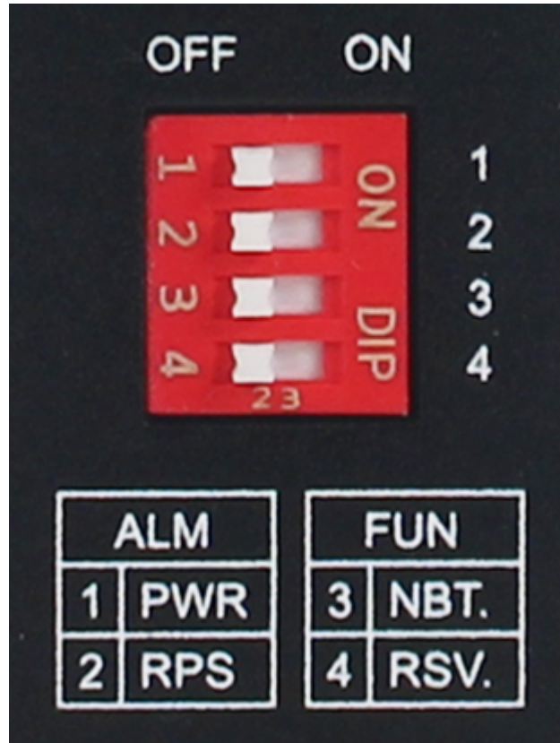
Abbildung 6: DIP-Schalter
