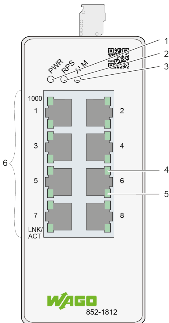
Abbildung 1: Frontansicht des Lean-Managed-Switches
