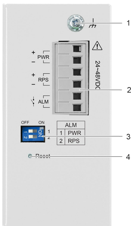
Abbildung 2: Draufsicht des Lean-Managed-Switches
