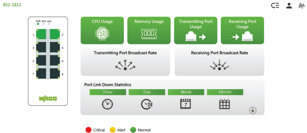
Abbildung 12: Dashboard
