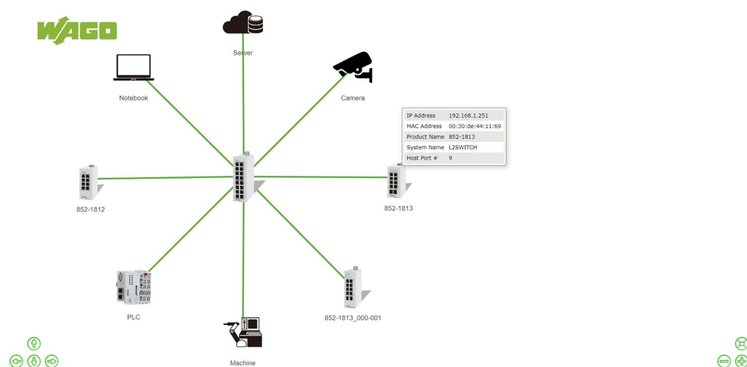
Abbildung 27: Topologiekarte – Verbindungsinformationen
