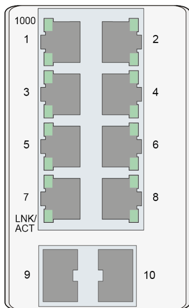
Abbildung 7: Anschluss-LEDs
