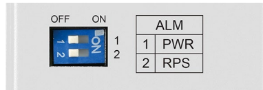
Abbildung 8: DIP-Schalter
