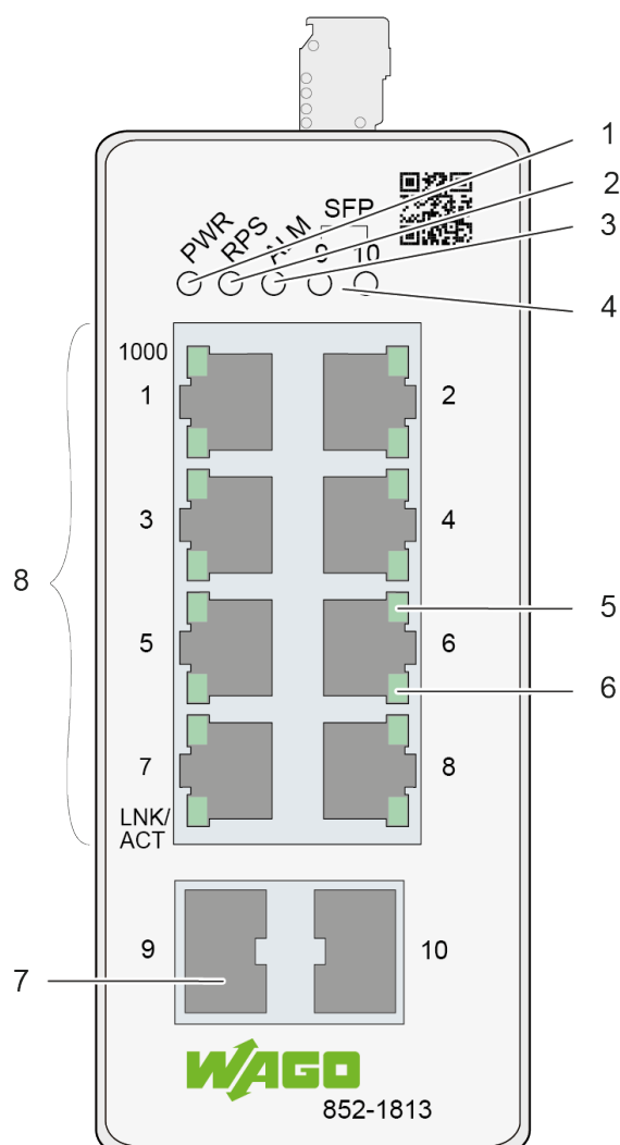
Abbildung 1: Frontansicht des Lean-Managed-Switches
