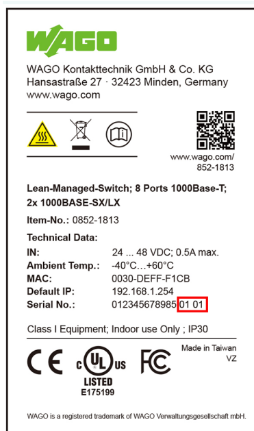
Abbildung 10: Aufkleber
