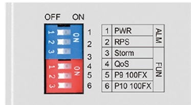
Abbildung 8: DIP-Schalter
