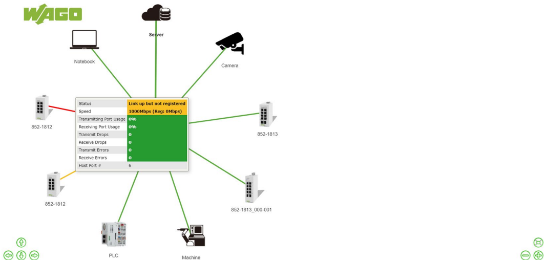
Abbildung 31: Topologiekarte – Verbindung nicht registriert
