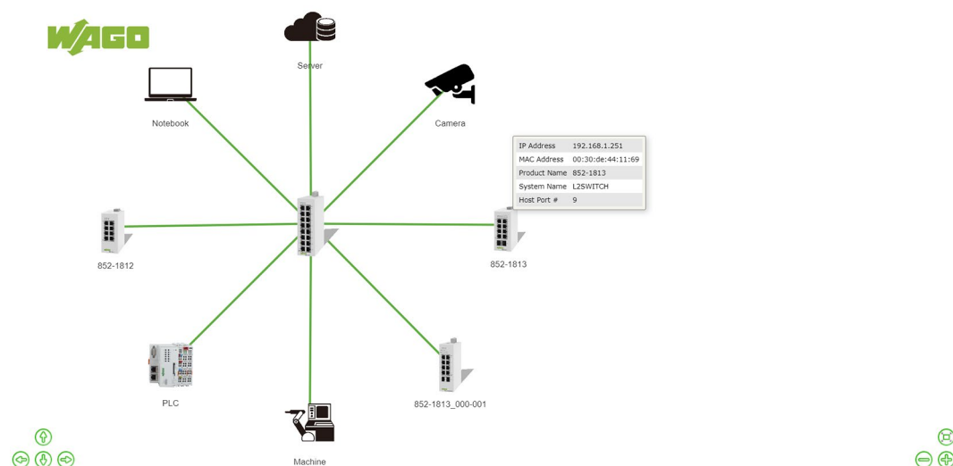
Abbildung 32: Topologiekarte – Verbindungsinformationen
