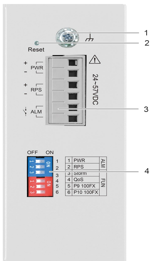
Abbildung 2: Draufsicht des Lean-Managed-Switches
