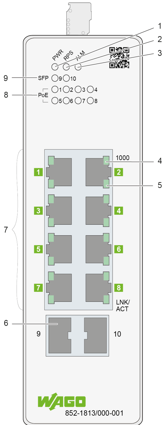
Abbildung 1: Frontansicht des Lean-Managed-Switches
