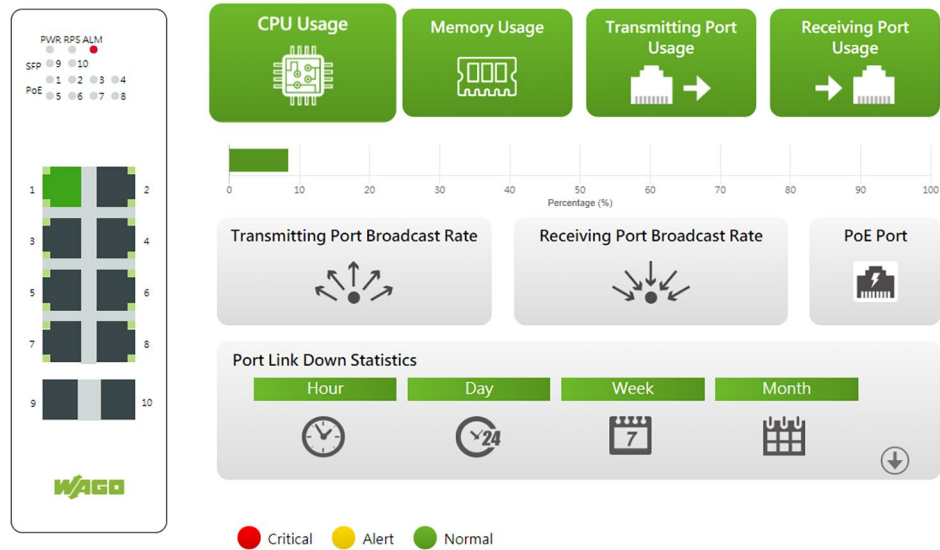
Abbildung 16: Dashboard
