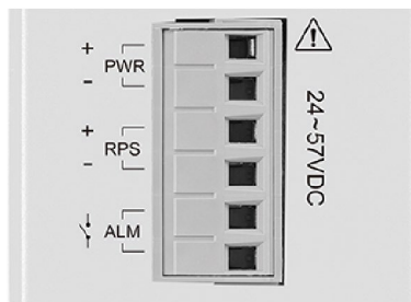
Abbildung 4: Anschluss Spannungsversorgung (PWR/RPS)
