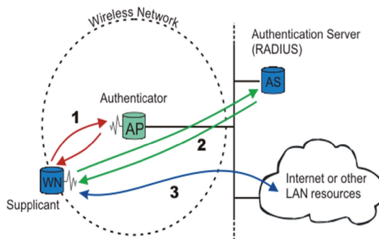
Abbildung 66: IEEE 802.1X
