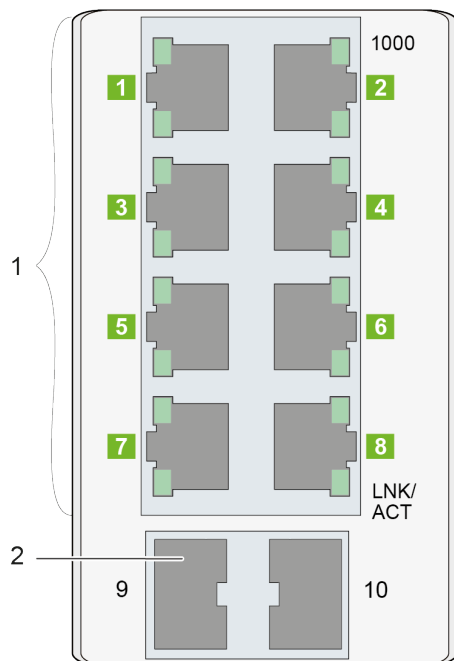
Abbildung 5: Netzwerkanschlüsse
