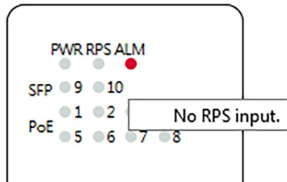
Abbildung 25: LED-Information
