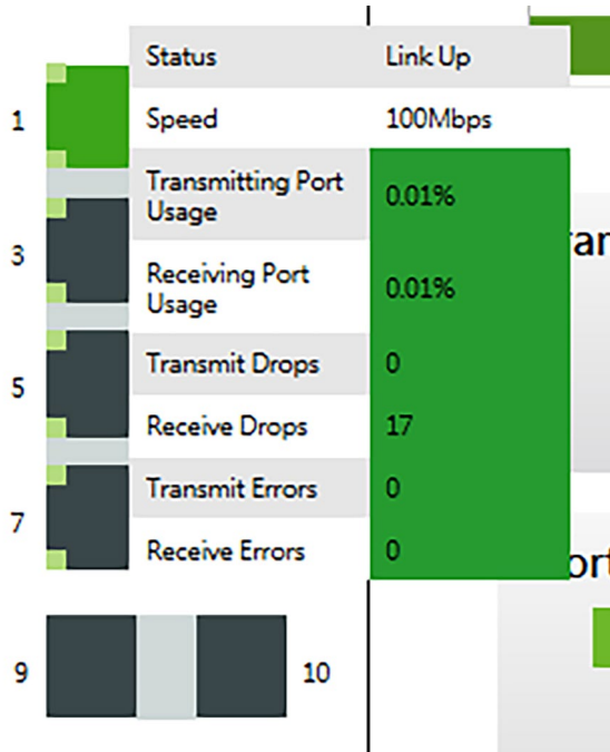
Abbildung 26: Anschlussinformation je Port (Beispiel)
