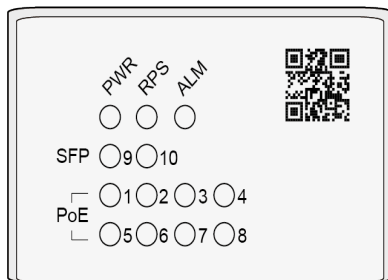
Abbildung 6: Geräte-LEDs
