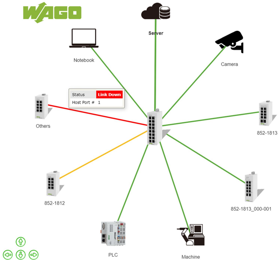
Abbildung 30: Topologiekarte – unterbrochene Verbindung an Port 1
