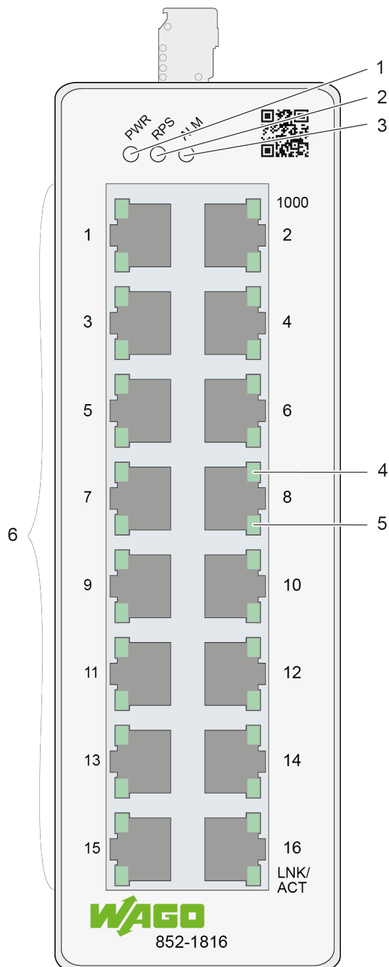
Abbildung 1: Frontansicht des Lean-Managed-Switches
