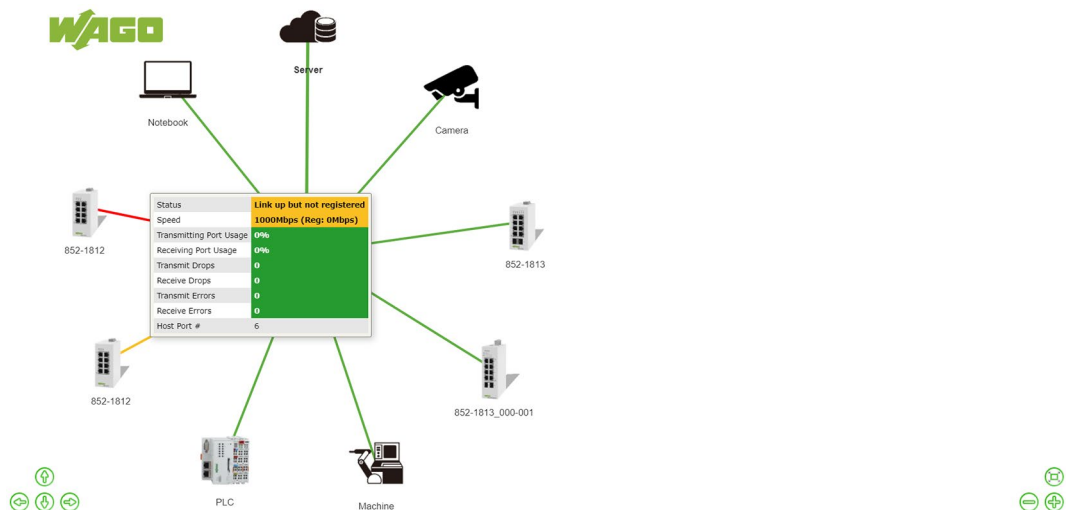
Abbildung 26: Topologiekarte – Verbindung nicht registriert
