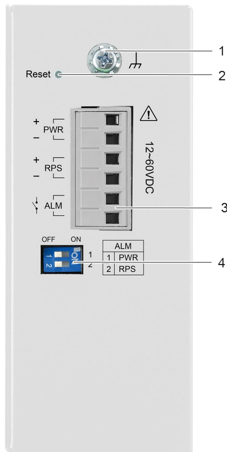
Abbildung 2: Draufsicht des Lean-Managed-Switches
