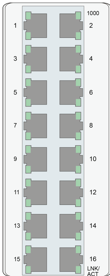
Abbildung 7: Anschluss-LEDs
