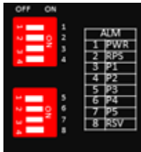
Ilustracja 6: Mikroprzełączniki DIP
