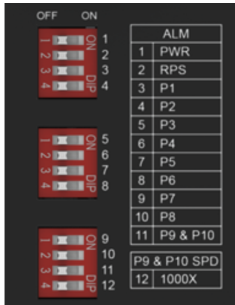
Ilustracja 6: Mikroprzełączniki DIP
