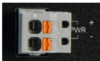
Ilustracja 3: Przyłącze zasilania
