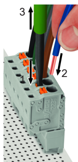
Ilustracja 8: Podłączenie przewodu do zacisku Push-in CAGE CLAMP®
