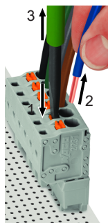
Ilustracja 9: Demontaż przewodu z zacisku Push-in CAGE CLAMP®
